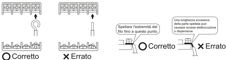
Spellatura del filo alla morsettiera
