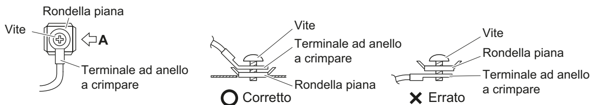
Vista nel senso della freccia A
